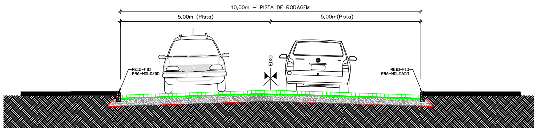
SEÇÃO TIPO DE BLOCO INTERTRAVADO - RUA MARECHAL EMÍLIO MALLET
